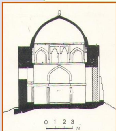
Оқ-Остона бобо мақбараси. Қирқим. X-XI асрлар.
