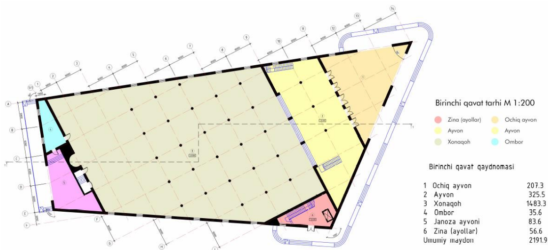
5-расм. Замонавий масжид тархи таклиф лойиҳаси. (Талабалар: И.Султонов, М.Шоюсупов. Раҳбар Ш.Бобоёрова).
