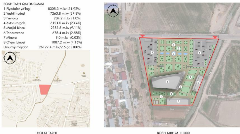
4-расм. Замонавий масжид бош тарх таклиф лойиҳаси. (Талабалар: И.Султонов, М.Шоюсупов. Раҳбар Ш.Бобоёрова).
